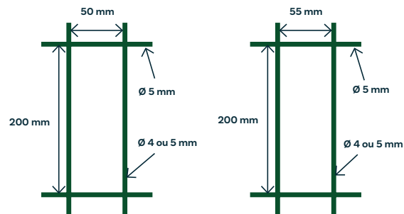
Dimensions des panneaux compatibles
